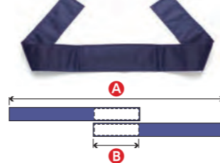
マジックシートベルト(1台分) MP22820A16-00(A16：紺) ¥4,350 部品価格オープン価格 寸法/A 70×920mm B マジック部 200mm
